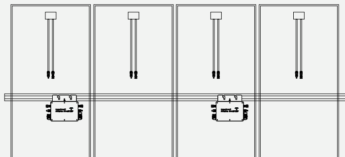
Abb.1 Installationseinbaulage des Mikrowechselrichters
